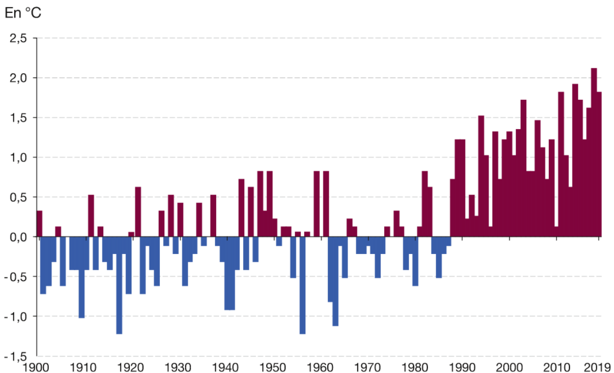
FIGURE 78 - TEMPERATURE EN FRANCE METROPOLITAINE DEPUIS 1901 - ECART A LA MOYENNE DE REFERENCE 1971-2000 Source : Météo France
