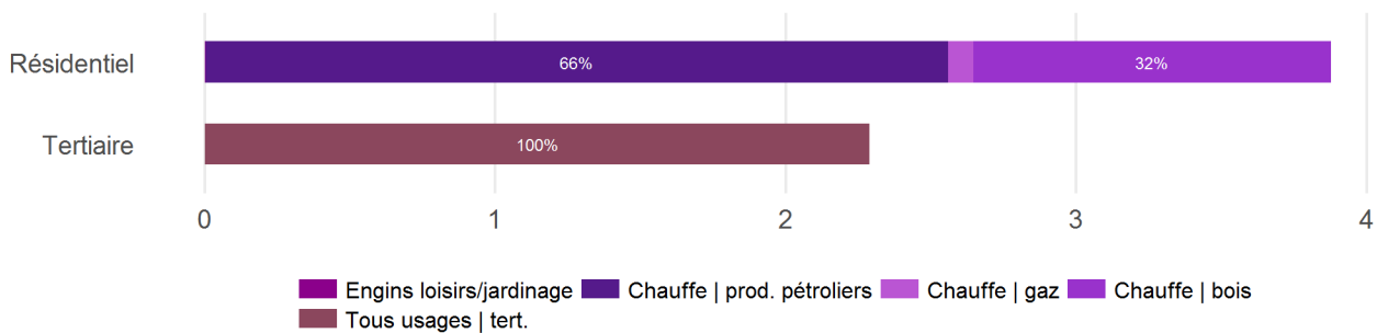
Figure 24 | CC des Rives de la Laurence – SO 2 , émissions des secteurs résidentiel et tertiaire, en tonnes
