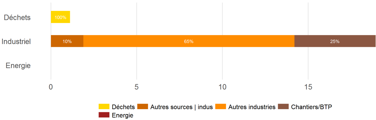
Figure 16 | CC des Rives de la Laurence – PM10, émissions des secteurs de l'énergie, de l'industrie et des déchets, en tonnes
