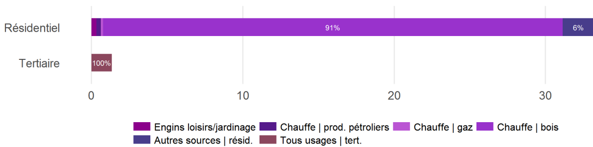
Figure 11 | CC des Rives de la Laurence – Émissions de PM2,5 des secteurs résidentiel et tertiaire, en tonnes
