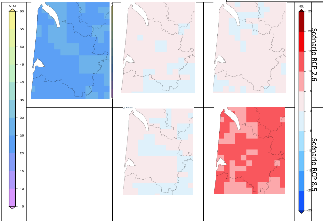
FIGURE 90- NOMBRE DE JOURS CONSECUTIFS AVEC MOINS DE 1 MM DE PRECIPITATIONS ESTIVALES POUR LA PERIODE DE REFERENCE 1976-2005 ET LES ECARTS A CETTE REFERENCE POUR LES SCENARIOS RCP.2.6 ET RCP 8.5, AUX HORIZONS 2021-2050 ET 2071-2100
