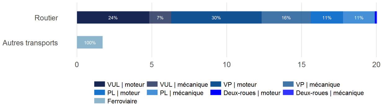
Figure 14 | CC des Rives de la Laurence – PM2,5, émissions du secteur des transports, en tonnes
