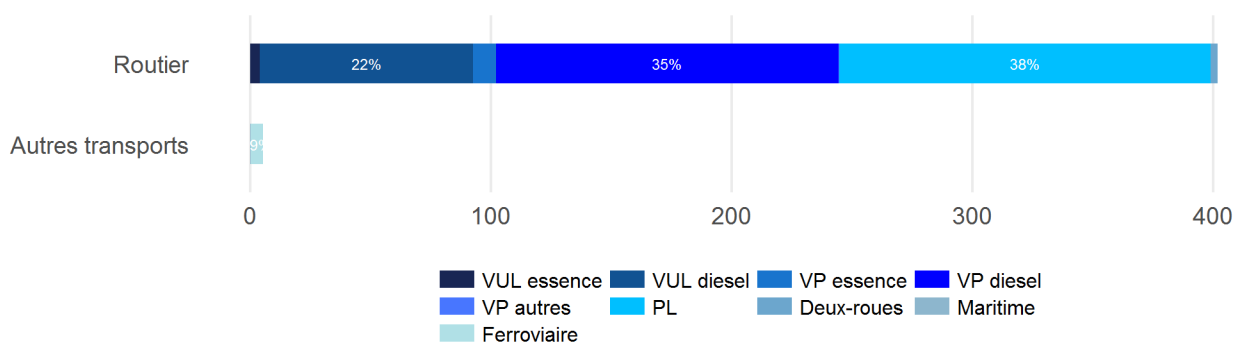
Figure 7 | CC des Rives de la Laurence – NOx, émissions du secteur des transports, en tonnes
