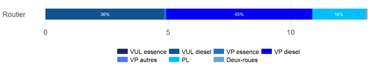
Figure 13 | CC des Rives de la Laurence – PM10, émissions liées à la combustion pour le transport routier, en tonnes
