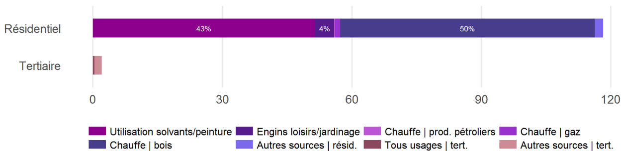
Figure 20 | CC des Rives de la Laurence – COVNM, émissions des secteurs résidentiel et tertiaire, en tonnes
