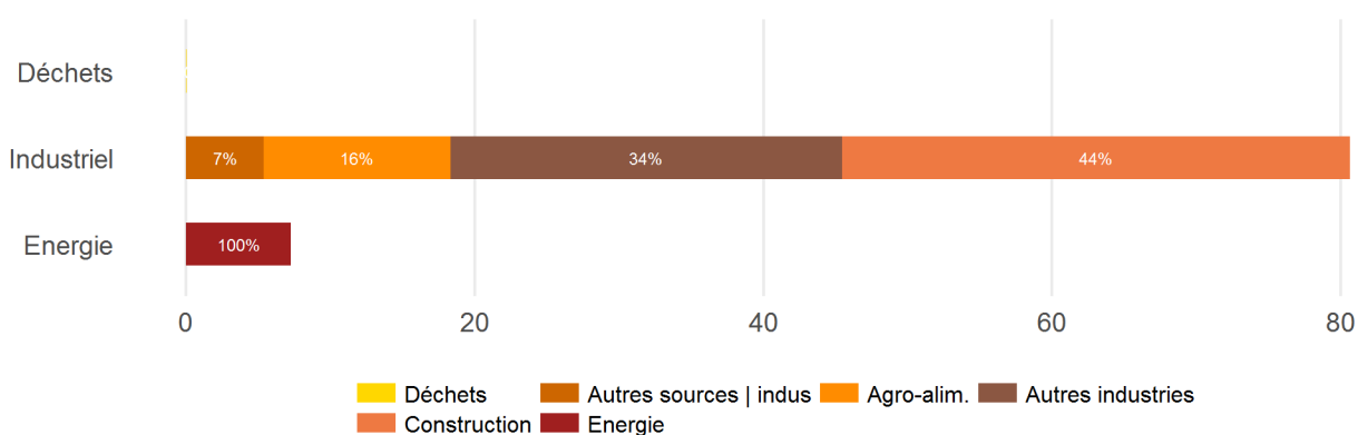
Figure 21 | CC des Rives de la Laurence – COVNM, émissions des secteurs de l'énergie, de l'industrie et des déchets, en tonnes
