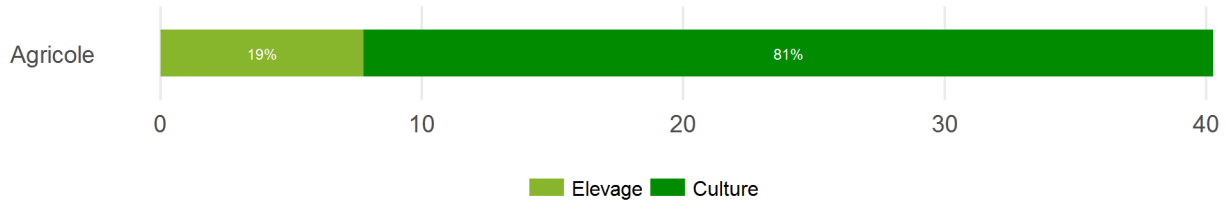
Figure 27 | CC des Rives de la Laurence – NH 3 , émissions du secteur agricole, en tonnes
