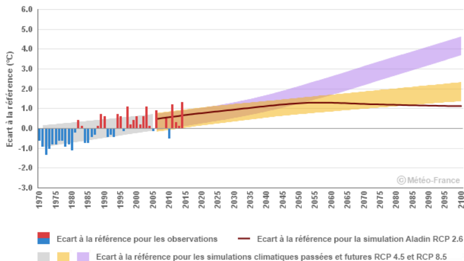
FIGURE 85 - TEMPERATURE MOYENNE ANNUELLE EN AQUITAINE : ECART A LA REFERENCE 1976-2005 OBSERVATIONS ET SIMULATIONS CLIMATIQUES POUR TROIS SCENARIOS D'EVOLUTION RCP2.6, 4.5 ET 8.5 Source : Météo France – Climat HD
