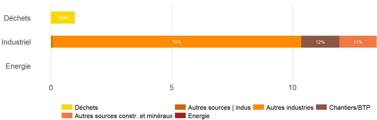
Figure 17 | CC des Rives de la Laurence – PM2,5, émissions des secteurs de l'énergie, de l'industrie et des déchets, en tonnes
