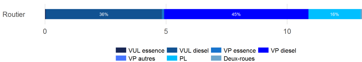
Figure 15 | CC des Rives de la Laurence – PM2,5, émissions liées à la combustion pour le transport routier, en tonnes
