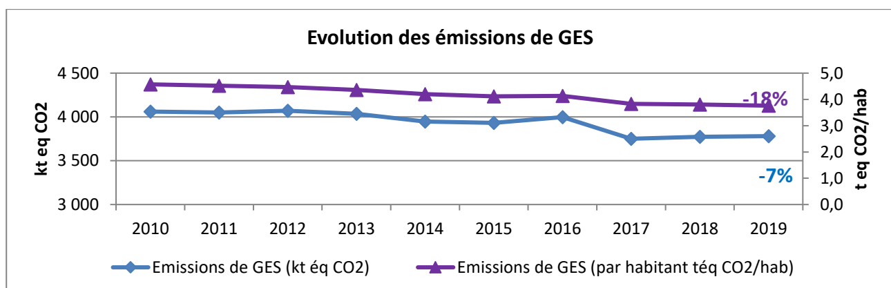
FIGURE 21 – EVOLUTIONS DES EMISSIONS DE GES ENTRE 2010 ET 2019
