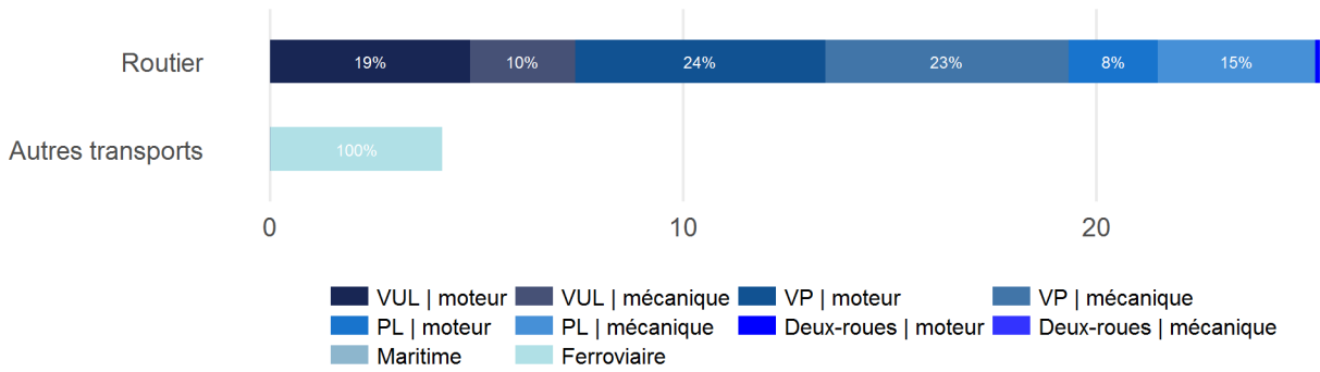
Figure 12 | CC des Rives de la Laurence – PM10, émissions du secteur des transports, en tonnes
